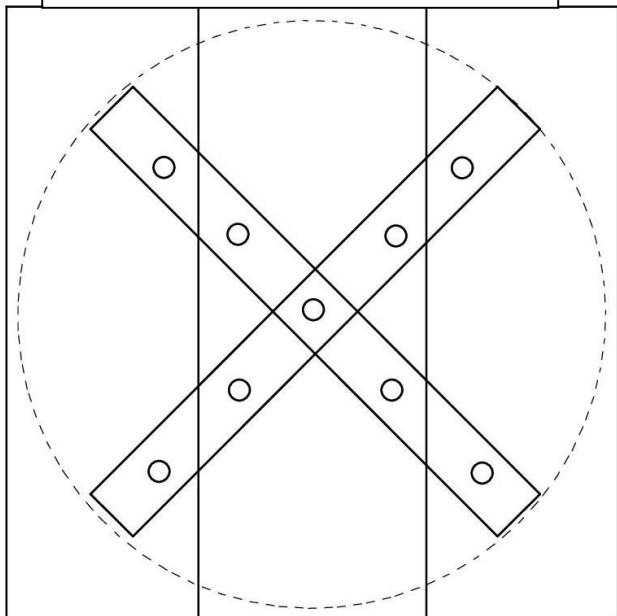
3枚の表板に均等に9カ所の木ねじ
